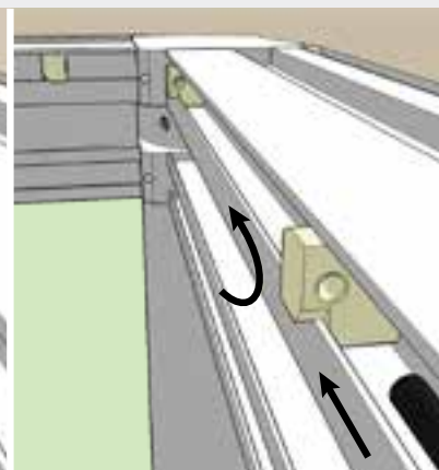
SYSTÈME D'ANCRAGE À LA TRAVERSE DU CHAPITEAU
