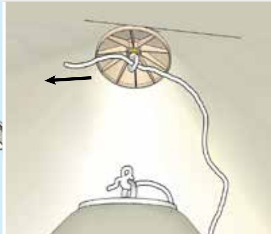
SYSTÈME D'ANCRAGE AU SOMMET DU CHAPITEAU
